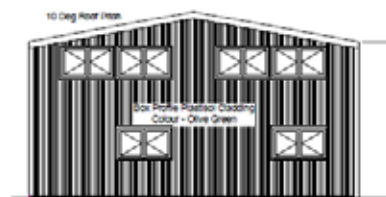
Right Elevation
